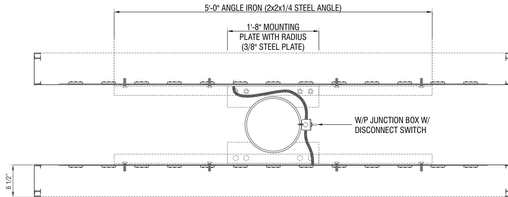
TOP VIEW SECTION SCALE: 1" = 1'-0"
