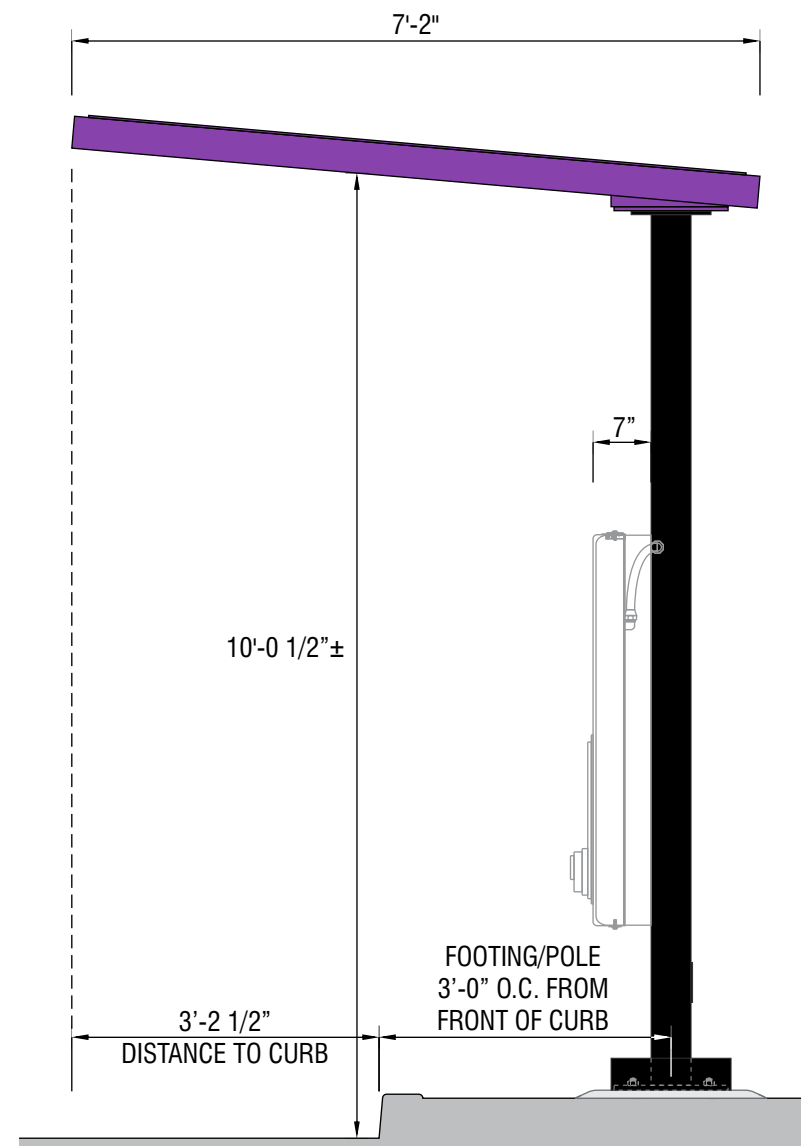
SIDE VIEW SCALE: 1/2" = 1'-0"
